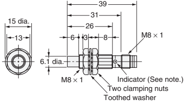
Fig. 29: E2E-X4MD□-M3G/E2E-X2ME□-M3/F□-M3
