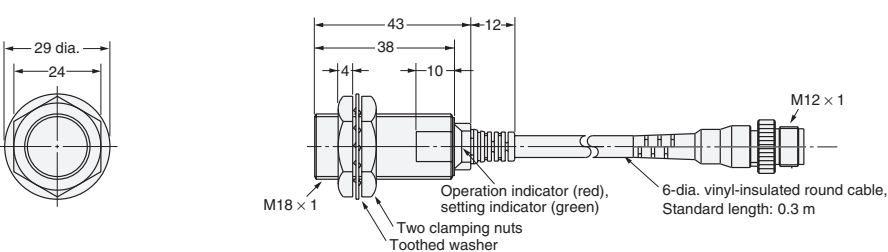
Fig. 32: E2E-X7D1-M1GJ E2E-X7D1-M1J-T
