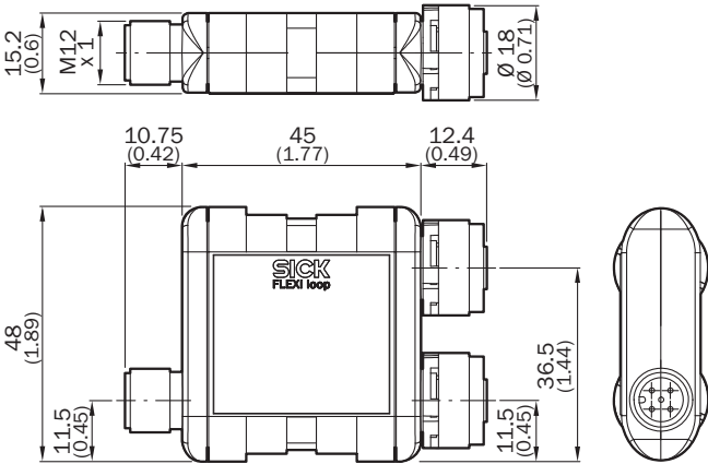
Размеры, мм
