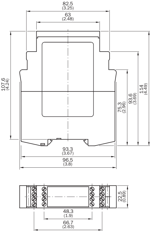
Размеры, мм
